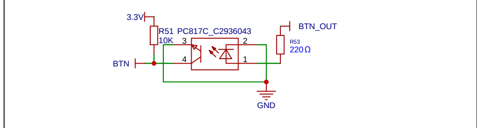
BUTTON DECOUPLER
