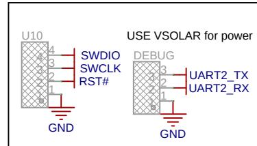
STLINK_PORT
