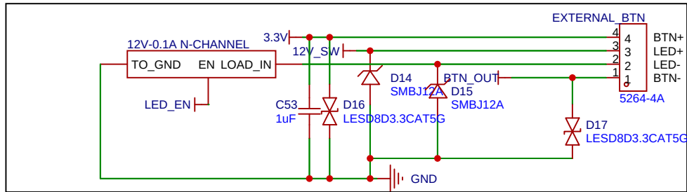
BUTTON DECOUPLER
